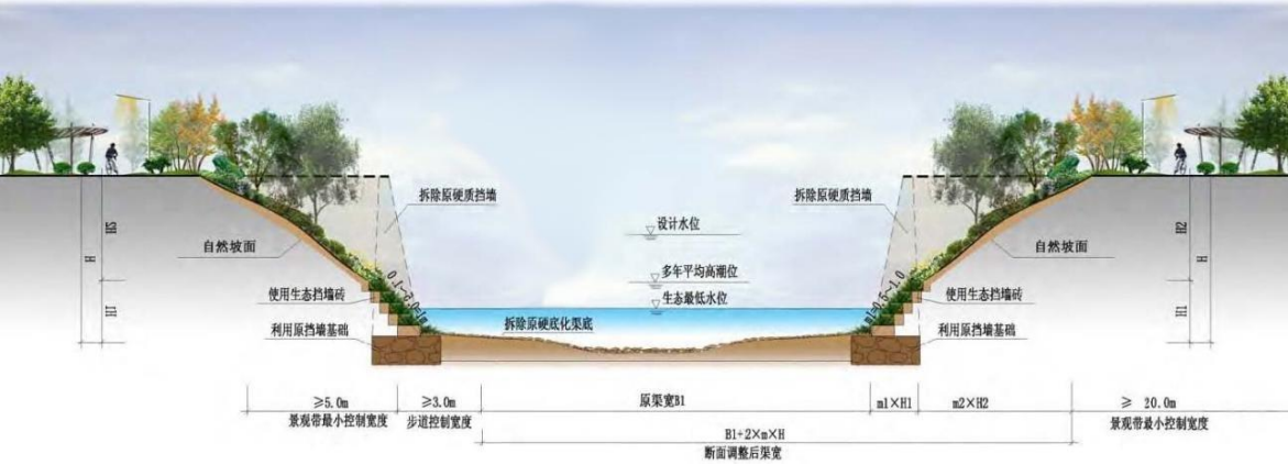
图64 10.2.5-7 现状河道改造示意图（双侧改造）
