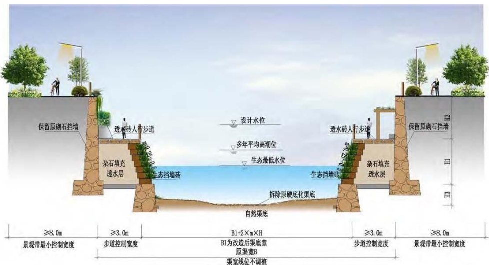
图60 10.2.5-3 现状河道改造示意图（两侧用地受限-打造亲水平台）
