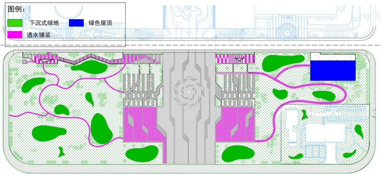
图36 10.2.2-4 LID 设施布置示意图
