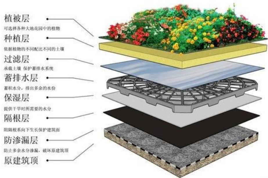
图28 10.2.1-6 绿色屋顶示意图
