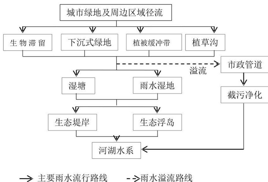
图4 城市绿地海绵城市系统构建示意图
