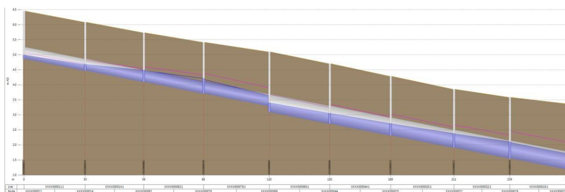
图57 10.2.4-5 5 年一遇降雨，雨水管道峰值纵断面示意图
