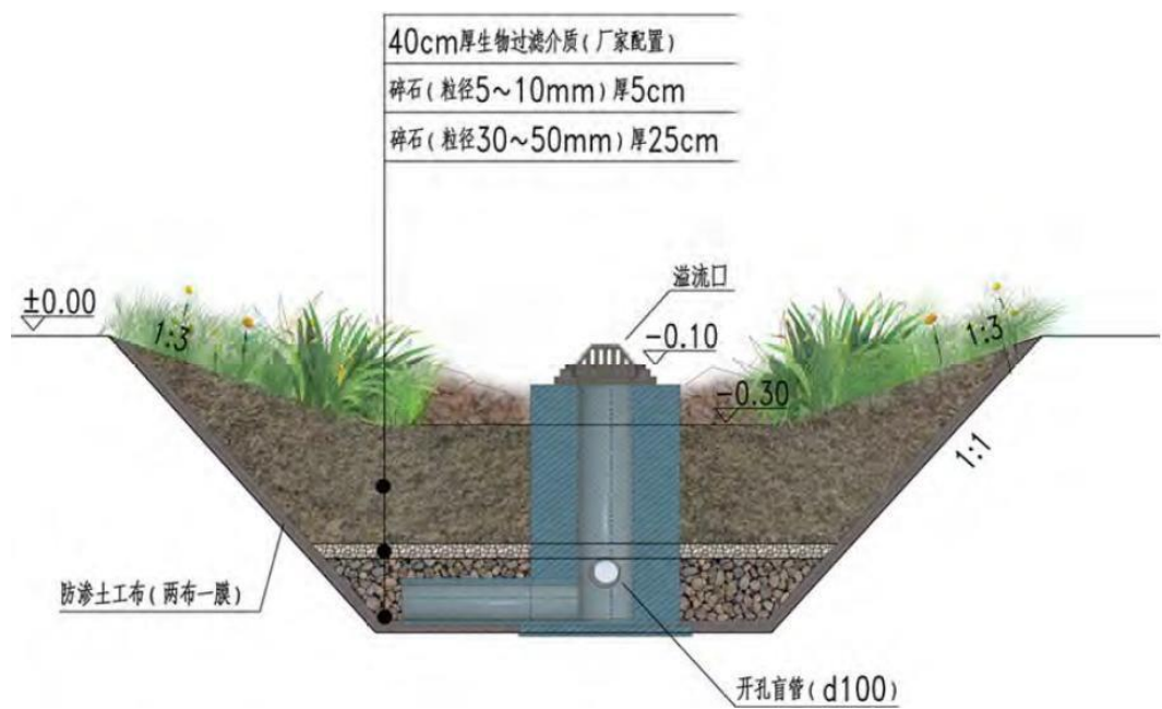
图30 10.2.1-8 下沉式绿地（雨水花园）示意图
