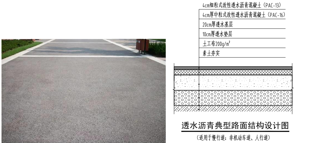
图8 透水沥青路面实景及结构参考图
