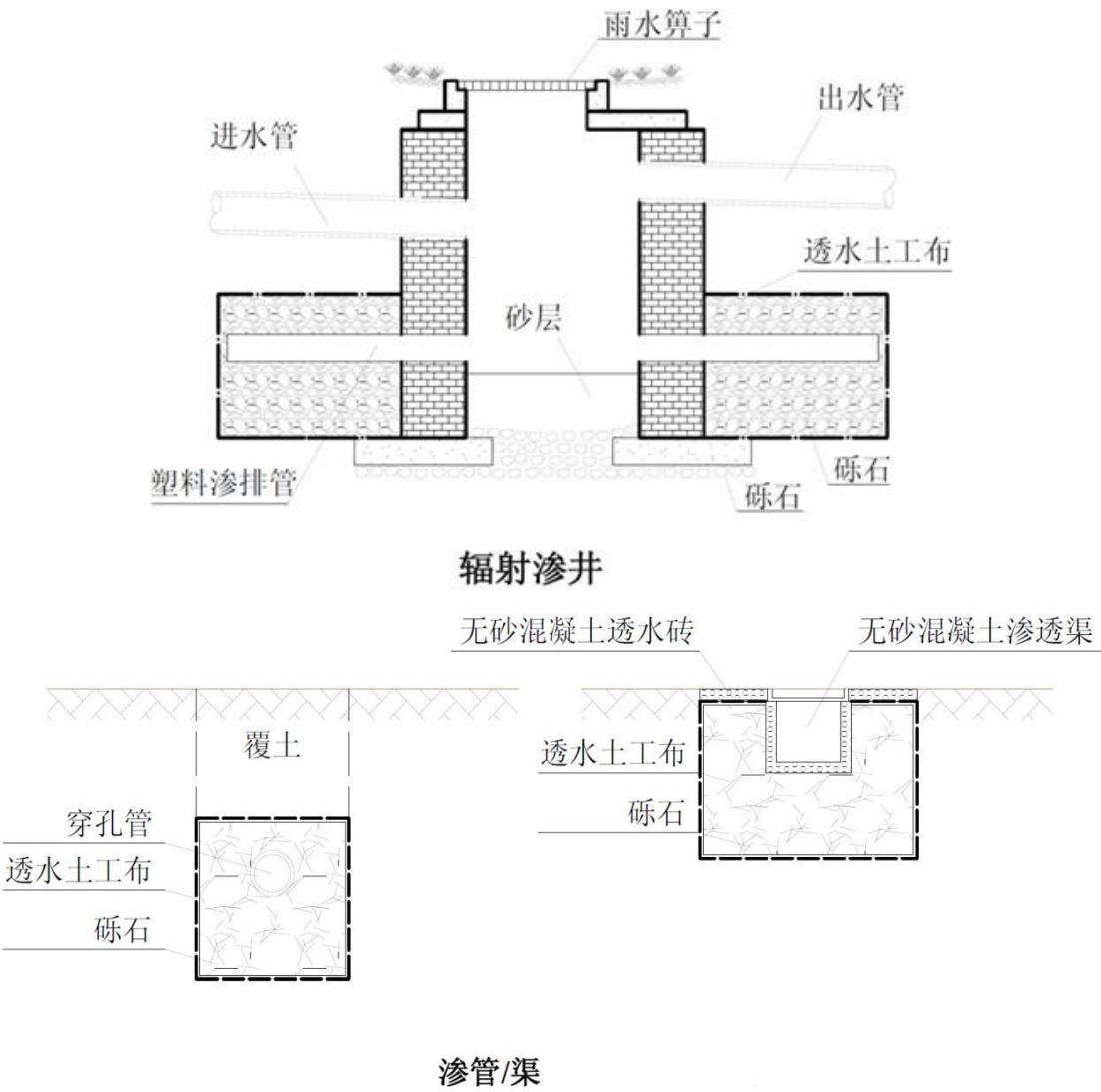
图17 渗井、渗管/渠结构参考图
