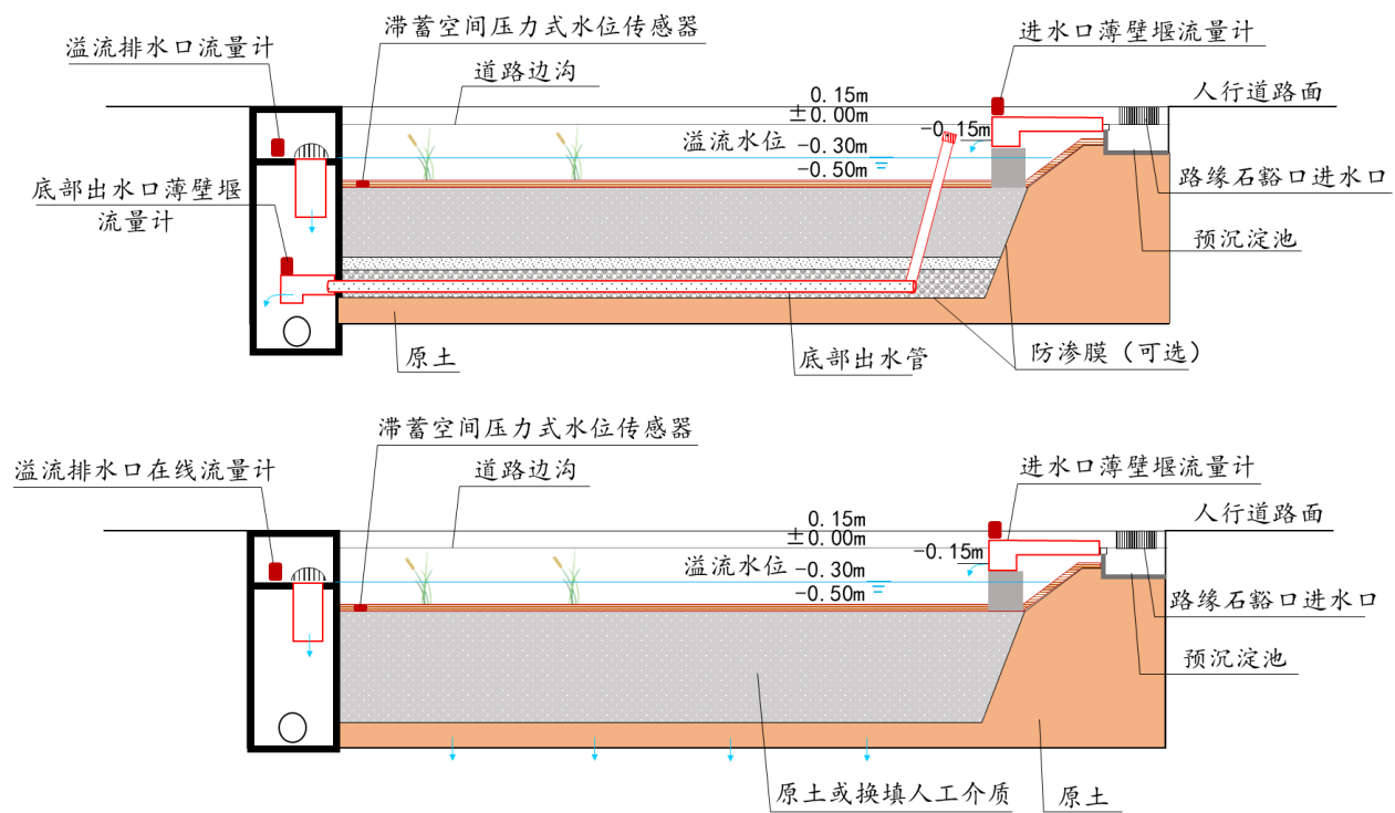
图21 生物滞留设施监测点布设（A-A断面图，上图设置底部出水口，下图无底部出水口）
