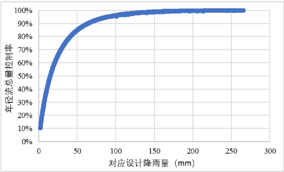
图1 江门市“雨水年径流总量控制率-设计降雨量”曲线图
