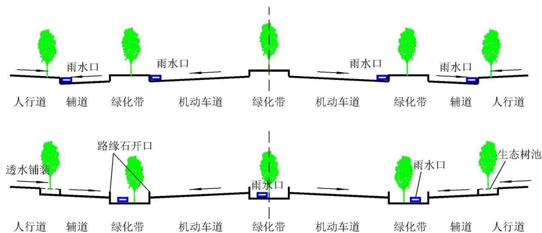
图40 10.2.3-1 传统道路（上）与低影响开发道路（下）排水示意图
