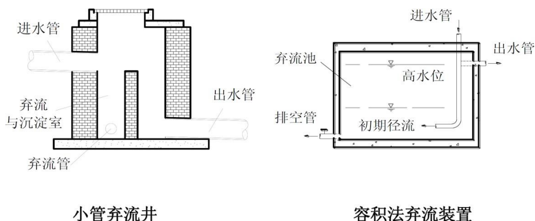
图16 初期雨水弃流结构参考图
