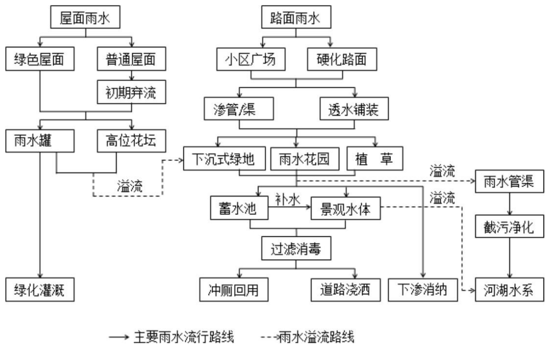
图2 建筑与小区海绵城市系统构建流程示意图
