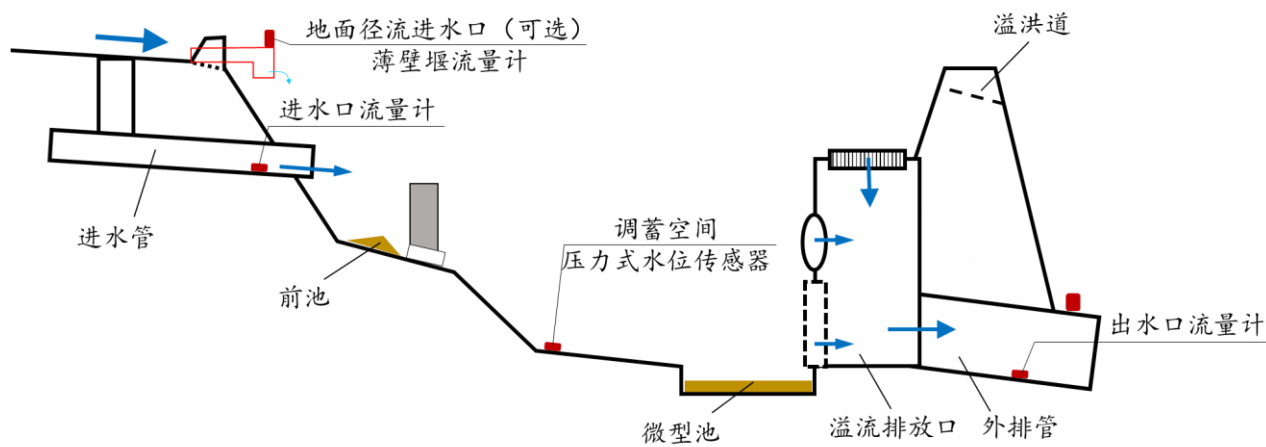
图22 调节塘监测点布设
