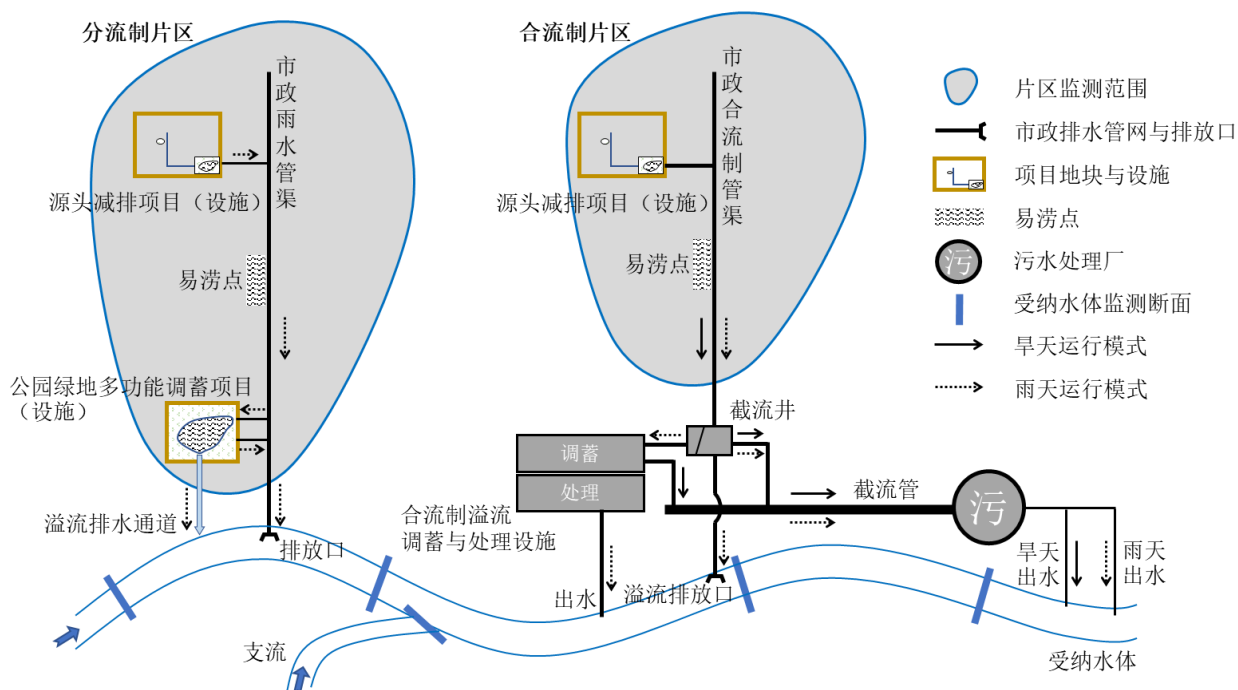
图7 片区监测范围、监测对象和监测点
