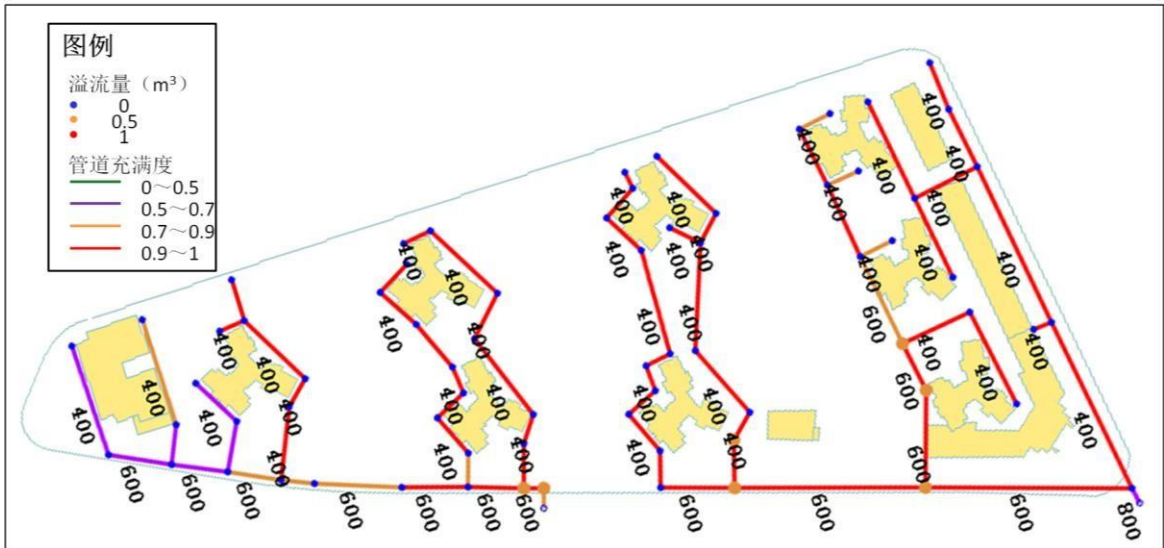
图31 10.2.1-9 30 年一遇内涝模拟分析图(布置 LID 设施前)
