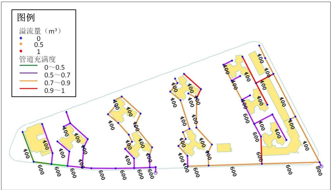
图32 10.2.1-10 30 年一遇内涝模拟分析图（布置 LID 设施后）
