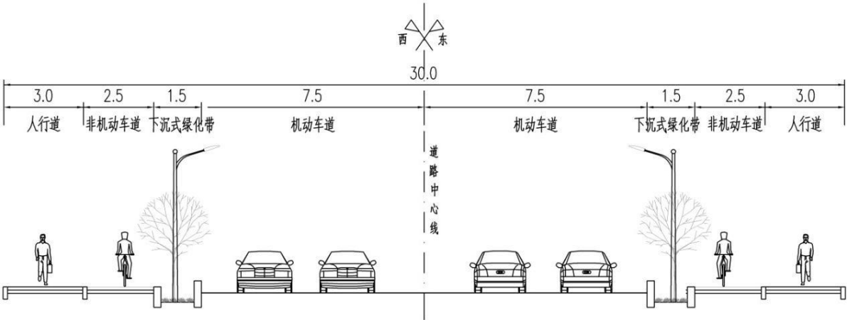
图52 10.2.4-1 道路横断面示意图
