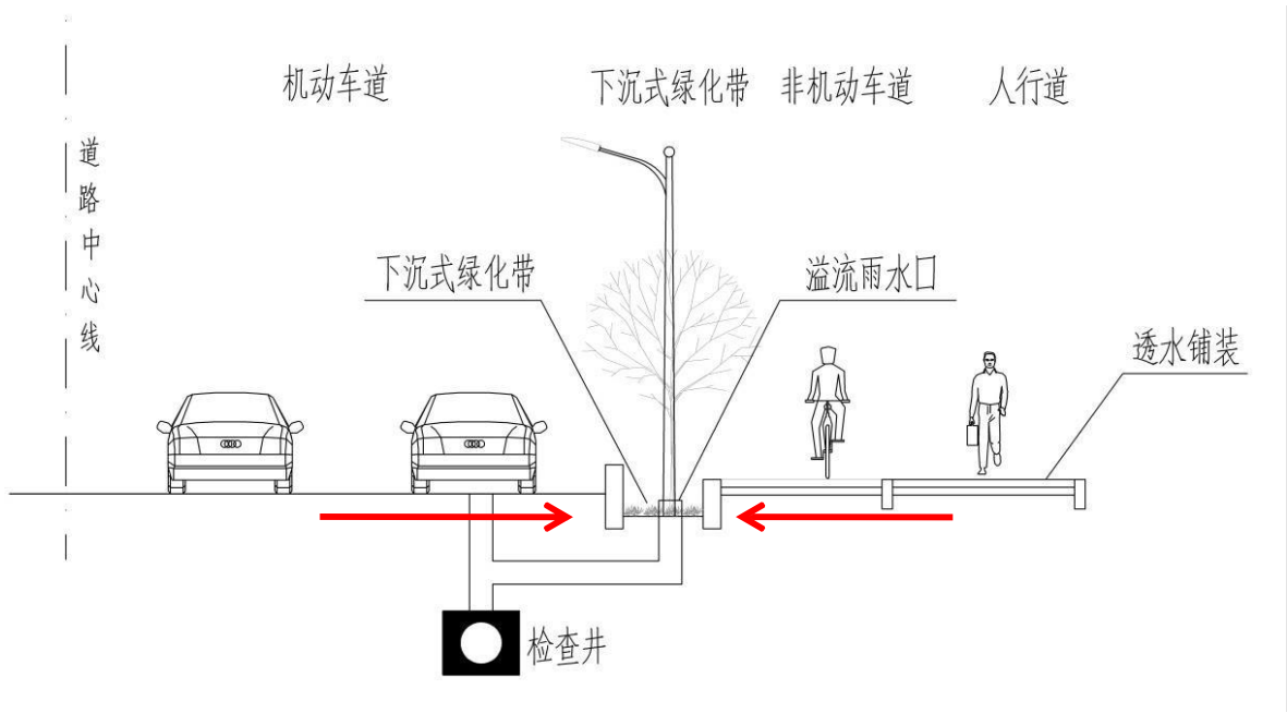
图55 10.2.4-4 道路横断面 LID 设施布置示意图
