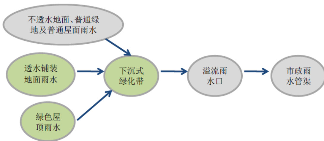
图35 10.2.2-3 技术路线示意图
