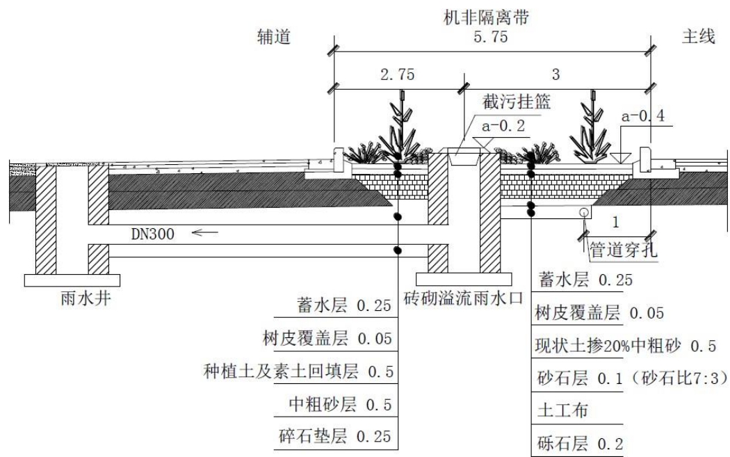
图11 道路下沉式绿地与植草沟结合实景及结构参考图
