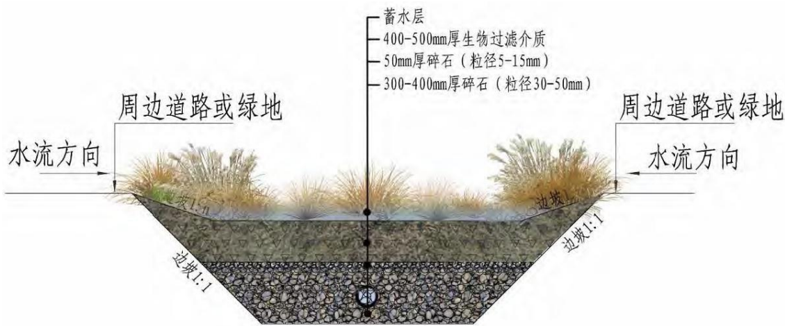
图37 10.2.2-5 雨水花园示意图
