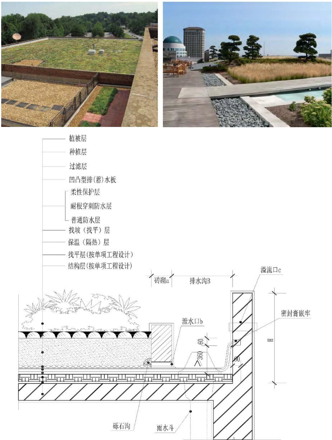
图14 绿色屋顶实景及结构参考图
