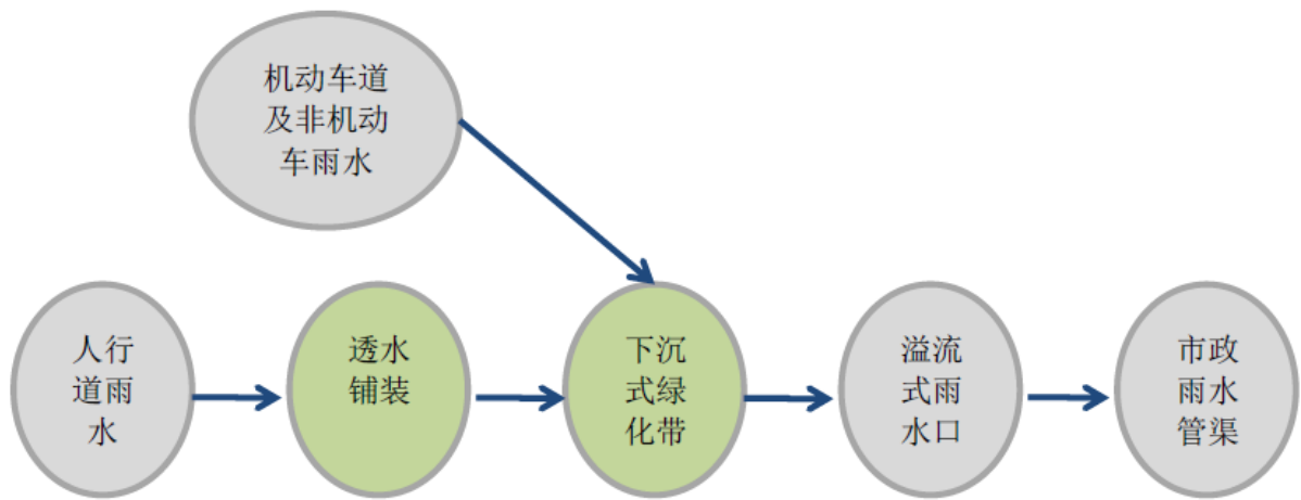
图54 10.2.4-3 技术路线示意图
