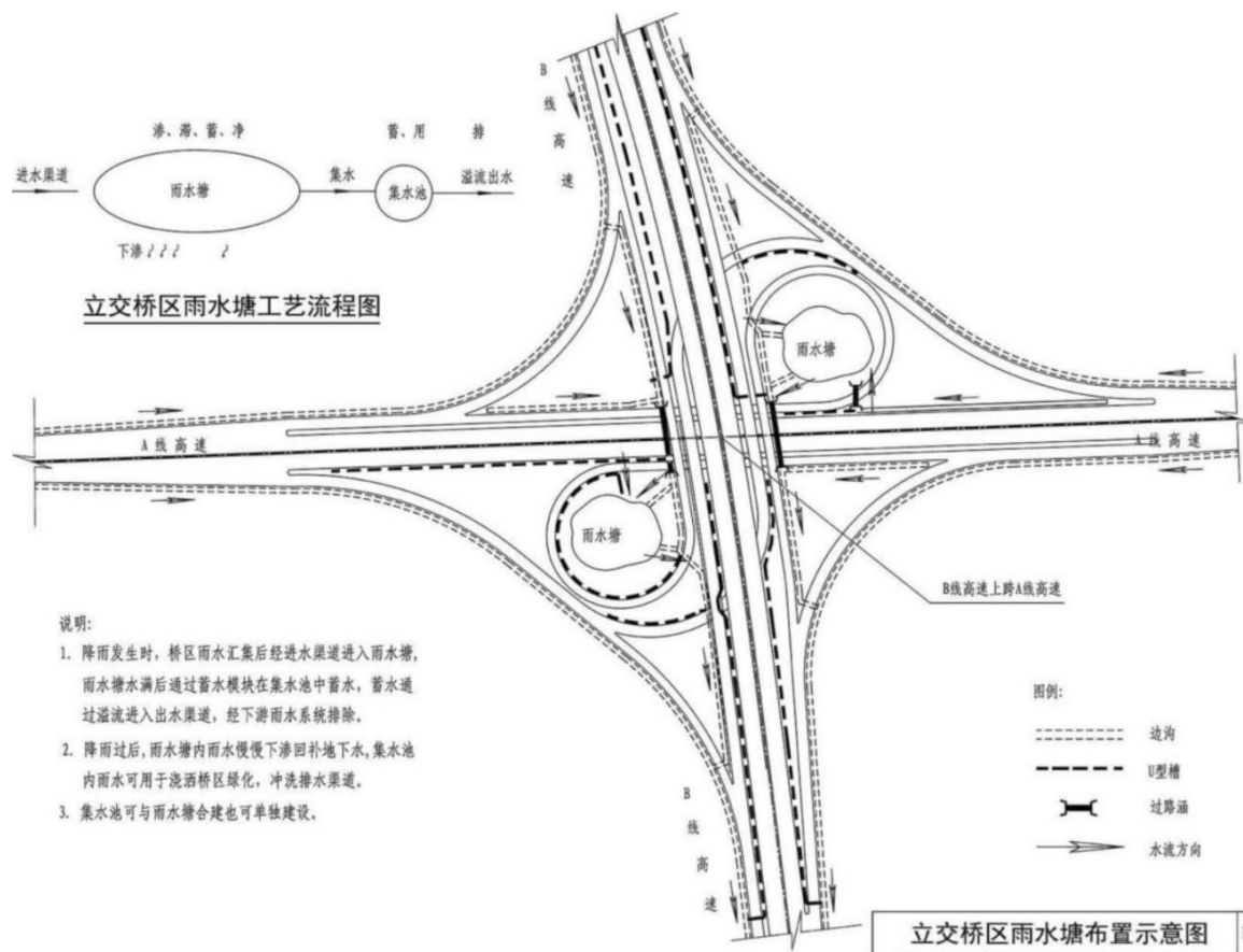
图50 10.2.3-11 立交桥区雨水塘布置示意图
