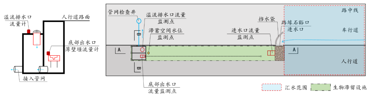
图20 生物滞留设施监测点布设（左图为B-B断面图，右图为平面图）
