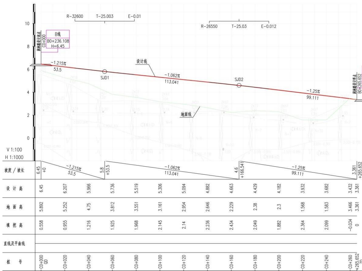
图53 10.2.4-2 道路纵断面示意图
