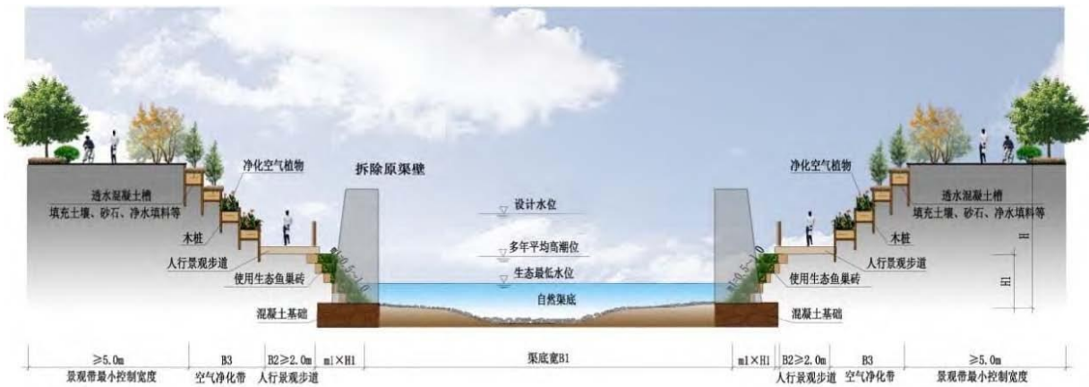
图65 10.2.5-8 现状河道改造示意图（双侧改造）
