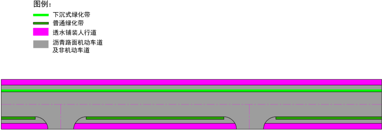
图56 10.2.4-5 道路平面 LID 设施布置示意图
