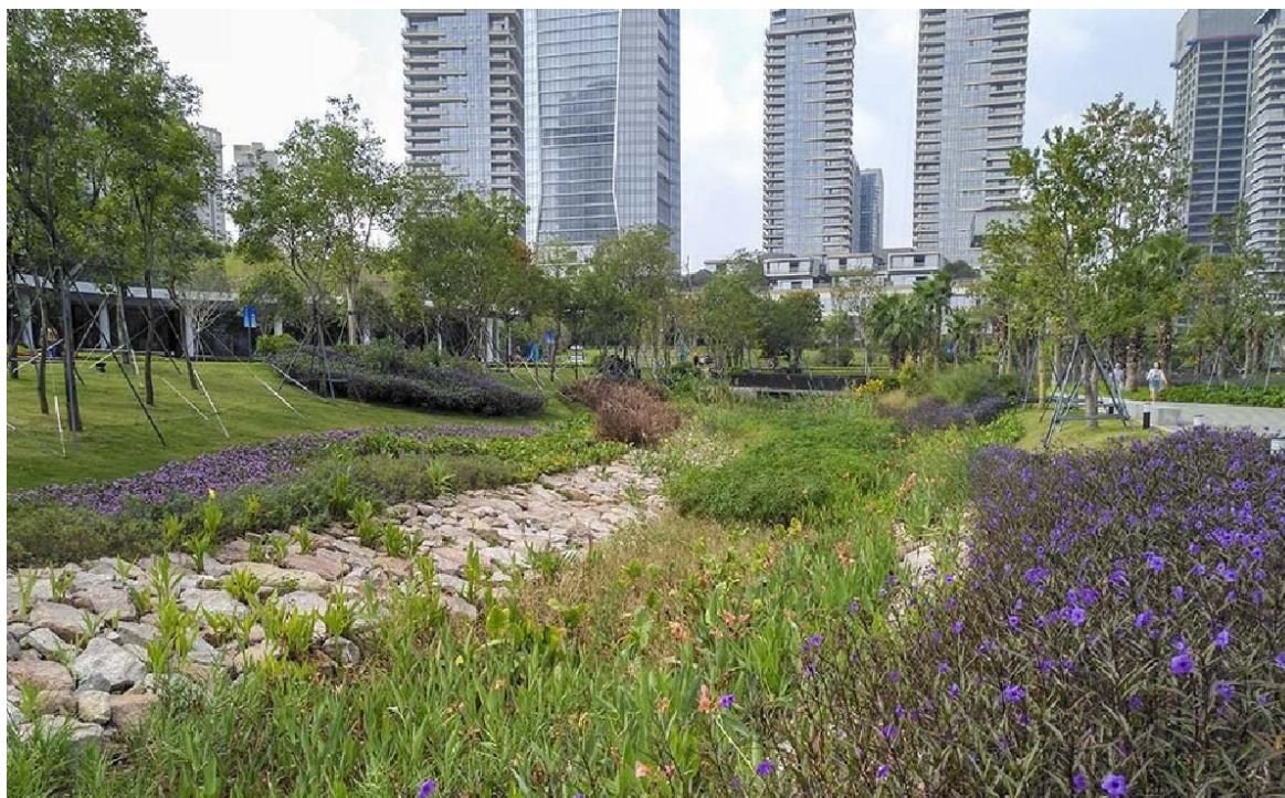
图12 生物滞留设施实景图
