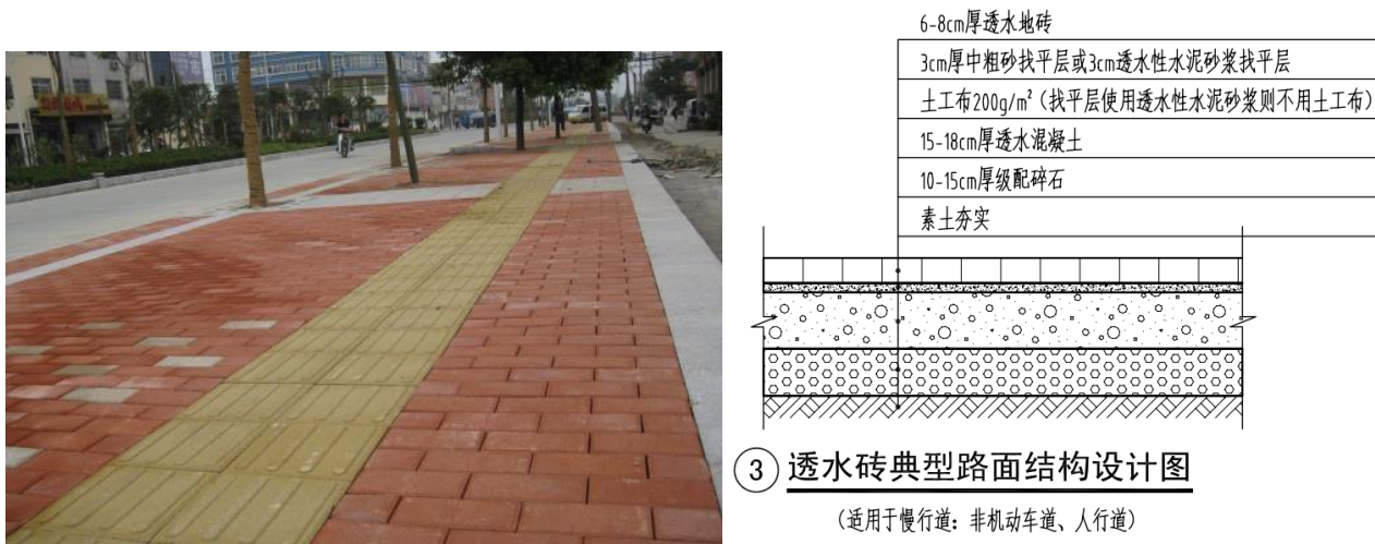
图9 透水人行道实景及结构参考图
