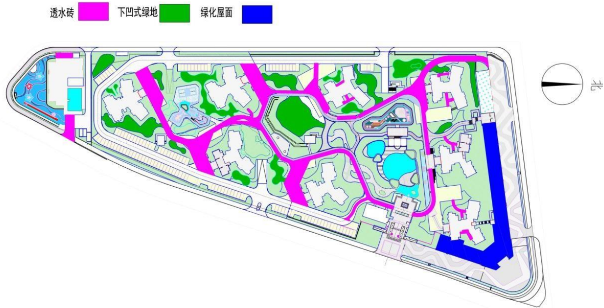
图27 10.2.1-5 LID 措施平面布置示意图
