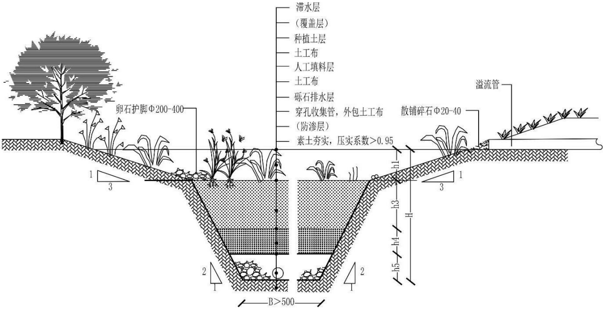
图13 雨水花园结构参考图
