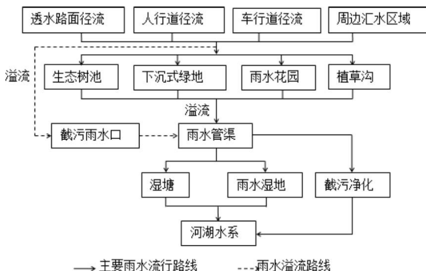
图3 城市道路海绵城市系统构建流程示意图
