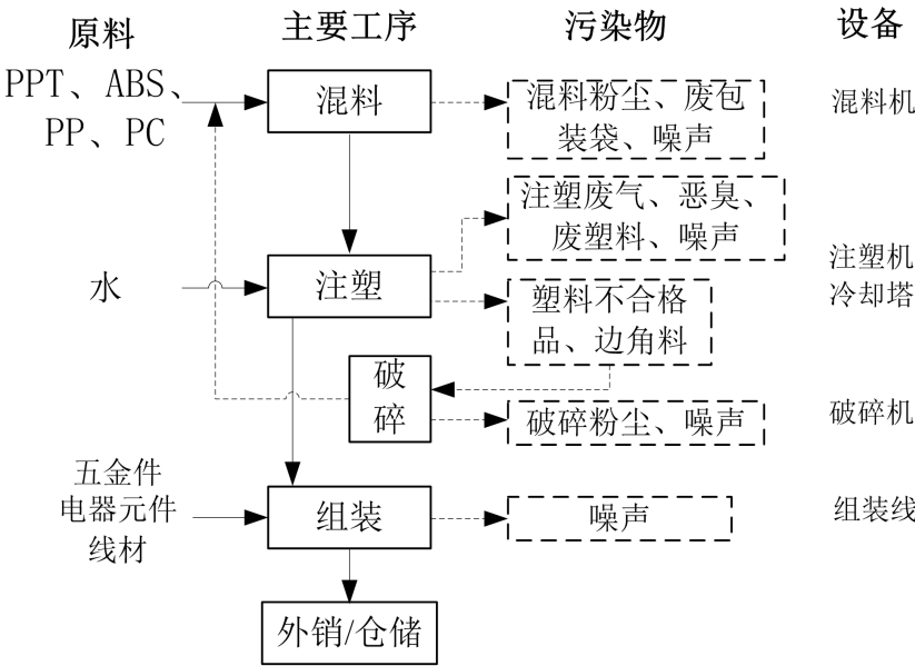
图 2-2 项目生产工艺流程图
