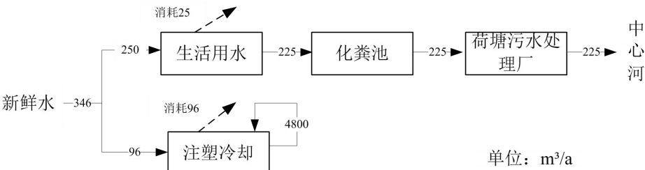
图2-1 项目水平衡图
