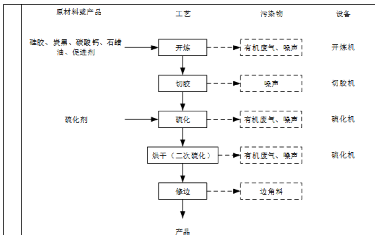
图 1. 密封圈生产工艺流程图
