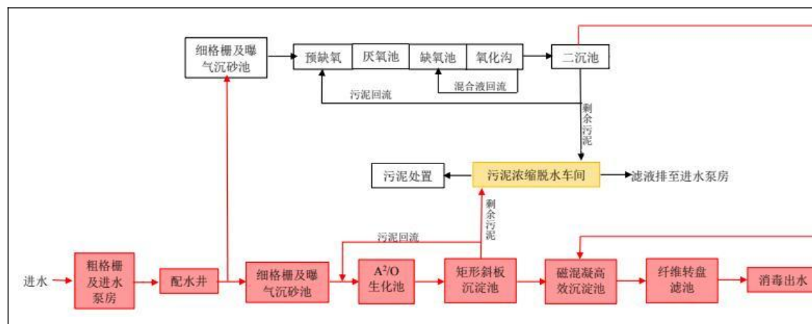
图 4-1 荷塘污水处理厂污水处理工艺流程图
