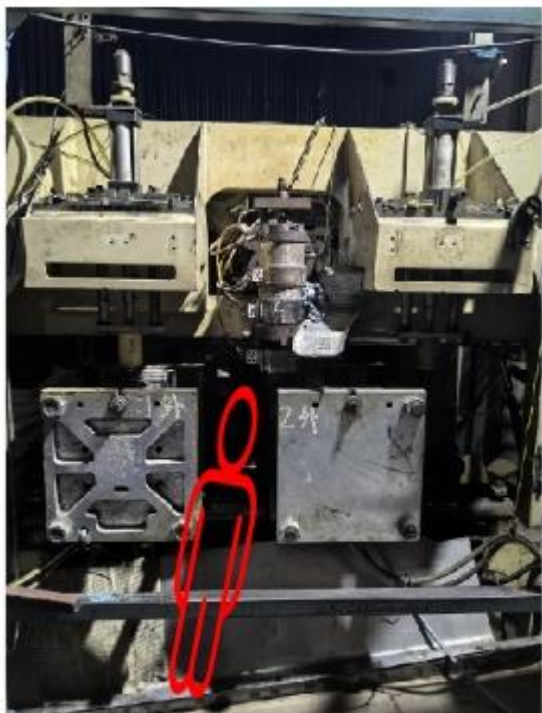
注塑设备事故点正面图
