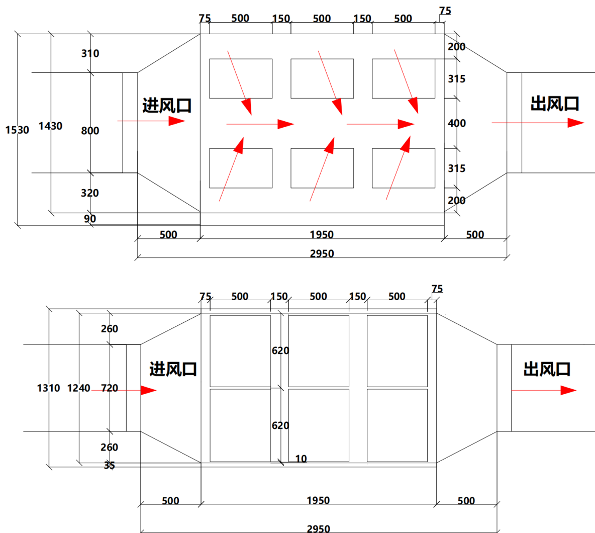
图 4-3 单级活性炭吸附装置结构示意图
