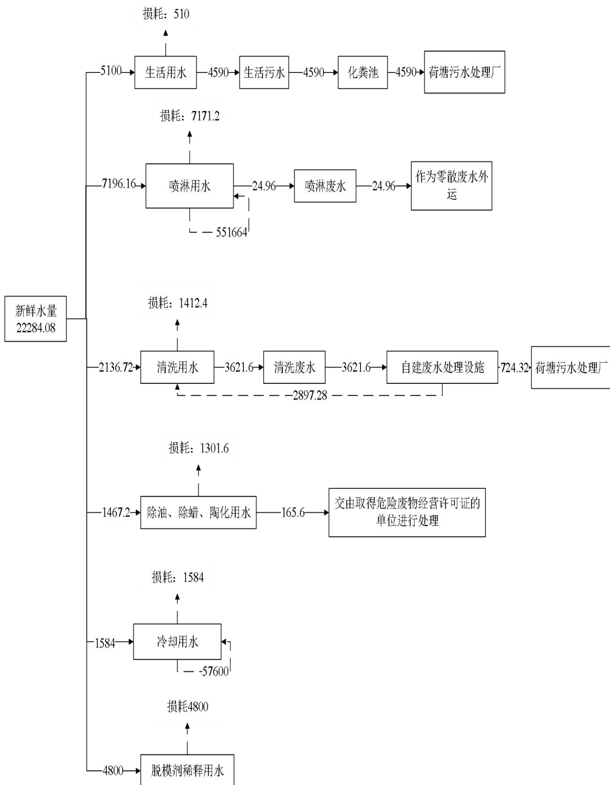
图 2-1 改建后全厂水平衡图（单位：t/a）
