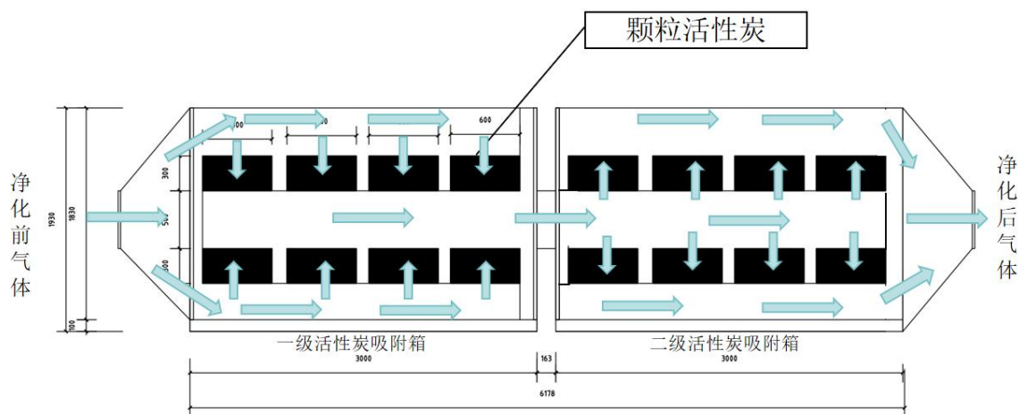
图4-3 活性炭箱体设计示意图
