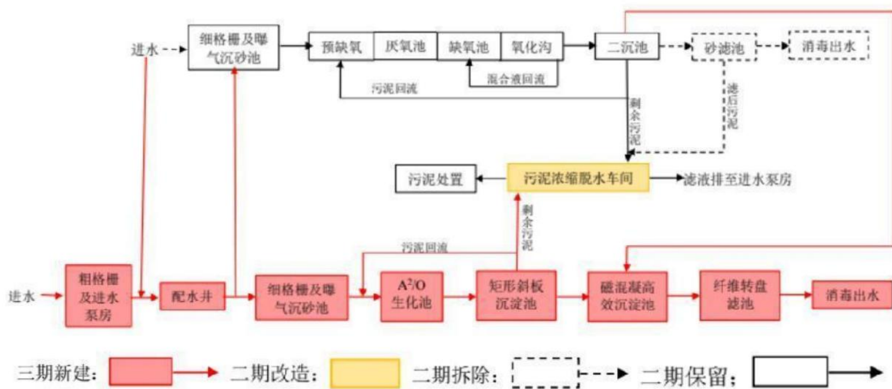
图 4-2 荷塘镇污水处理厂处理工艺
