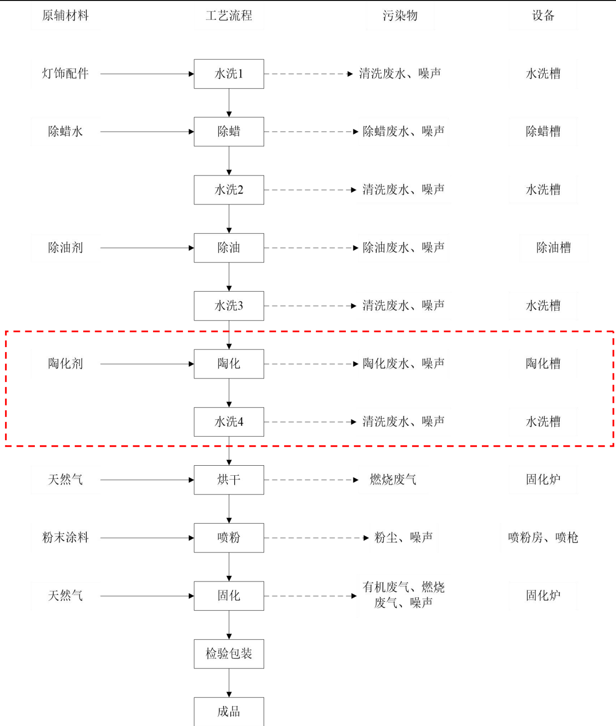
图 2-3 项目自动、手动清洗线生产工艺流程
