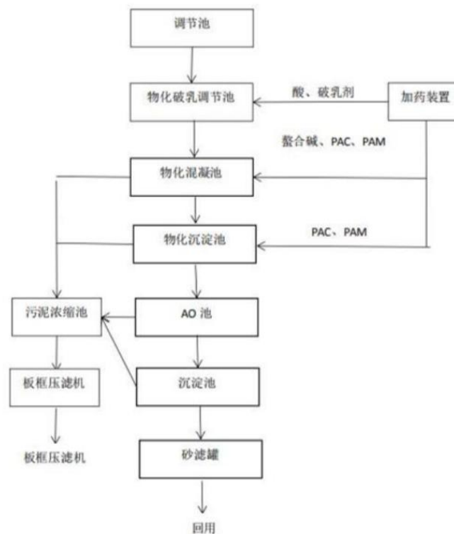
图4-1 本项目废水处理工艺流程图
