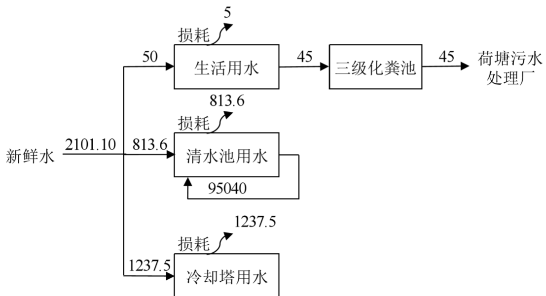
图 2-6 项目水平衡图 单位：t/a
