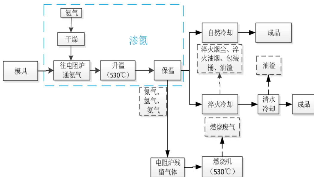
图 2-7 项目工艺流程及产污环节图
