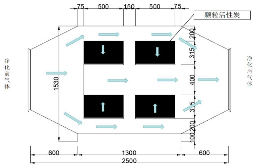
活性炭吸附箱剖面图 图 4-1 颗粒活性炭箱示意图
