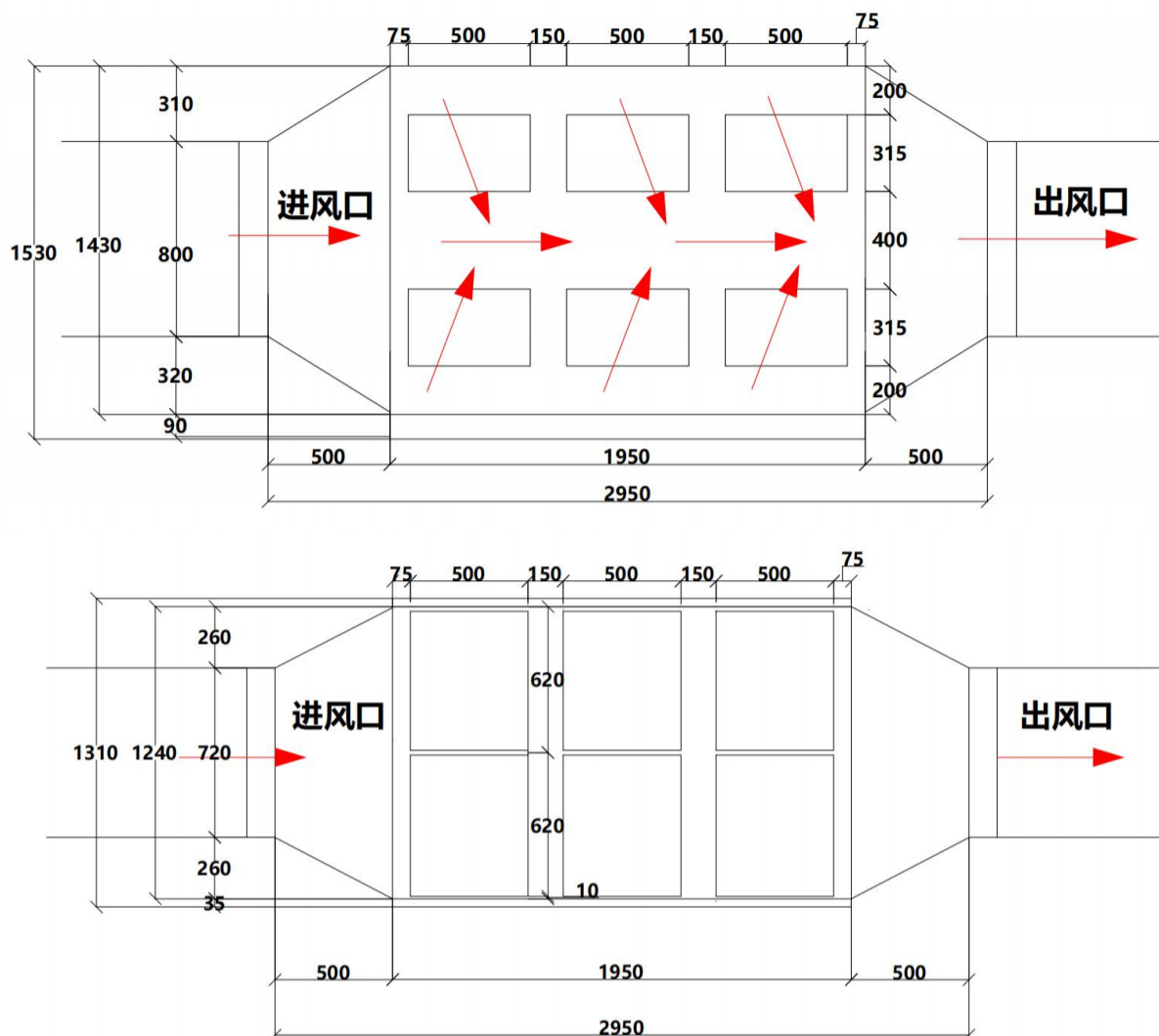
图 4-1 迁扩建项目单级活性炭箱结构图
