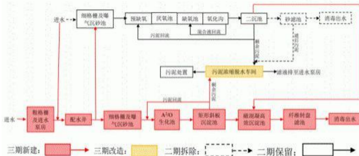
图4-2 荷塘污水处理厂工艺流程图
