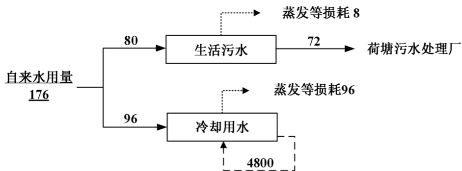
图 2-1 迁扩建后全厂水平衡图 单位：t/a
