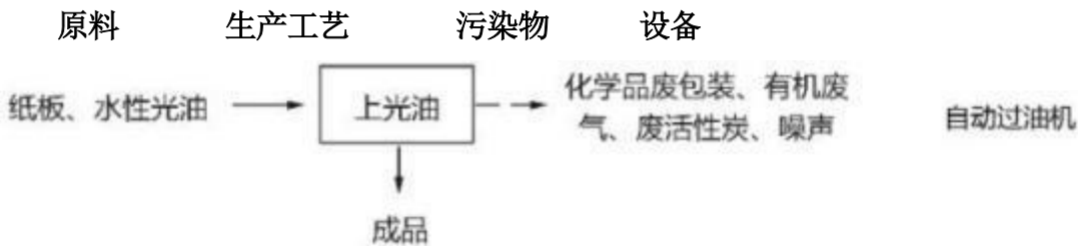
图 2-4 过水性光油纸制品生产工艺流程
