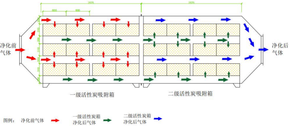
图4-1 活性炭箱设计图
