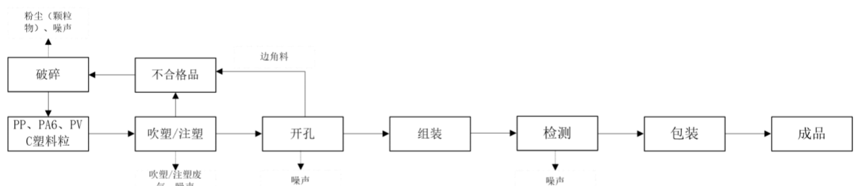
图 2-7 项目进气系统配件生产工艺流程
