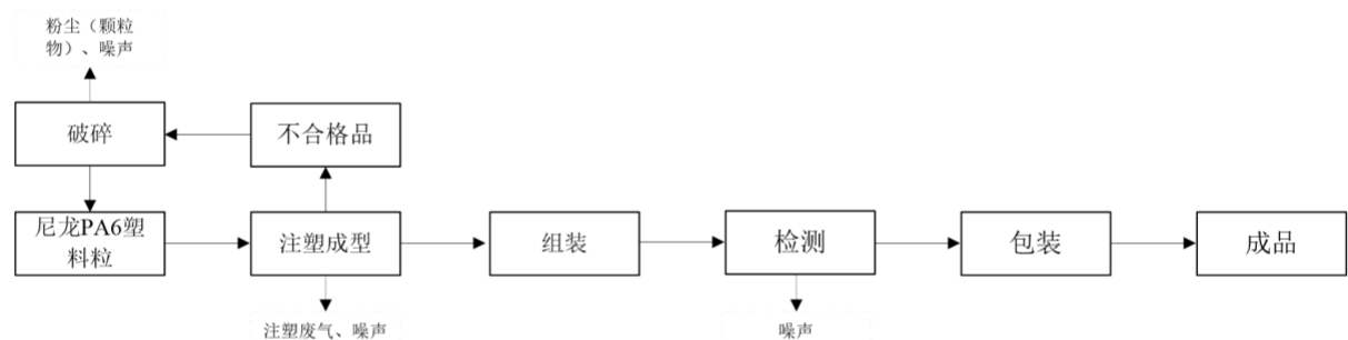
图 2-5 项目汽车通气管生产工艺流程
