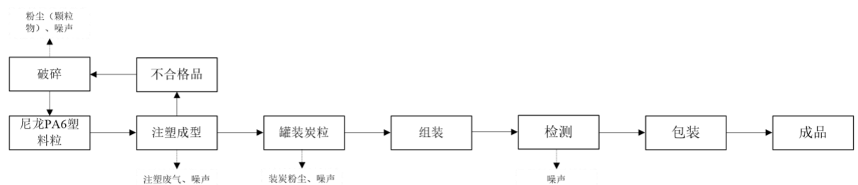
图 2-6 项目炭罐生产工艺流程
