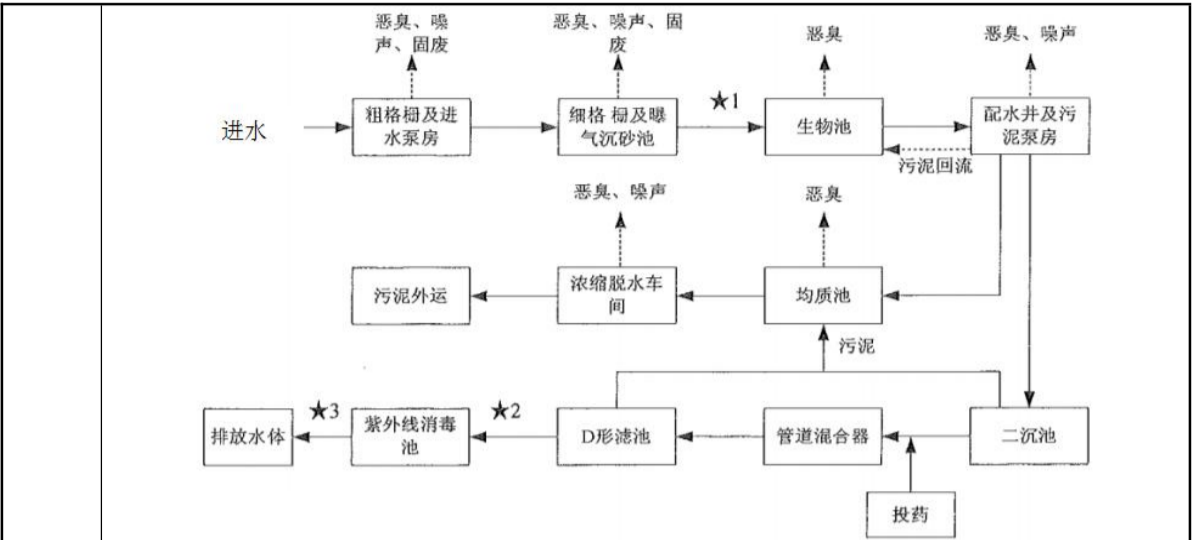
图 4-1 杜阮污水处理厂污水处理工艺流程图
