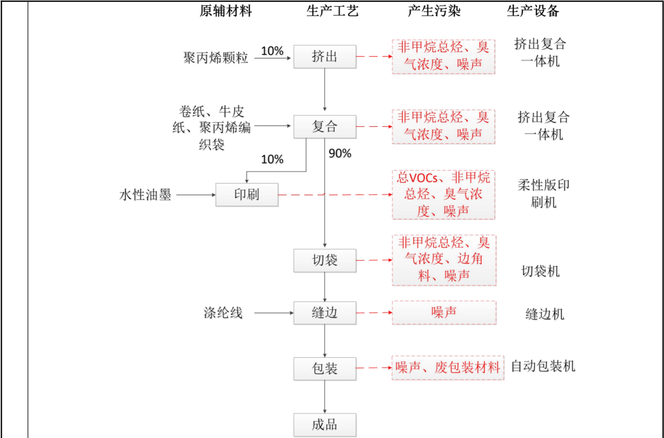
图 2-4 纸塑复合袋、编织袋生产工艺流程
