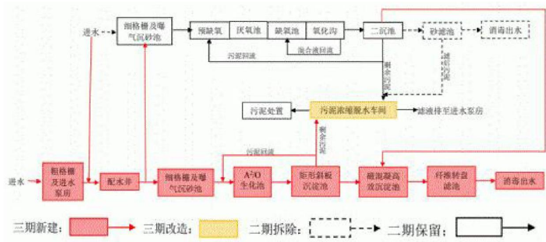
图 3. 荷塘污水处理厂污水处理工艺
