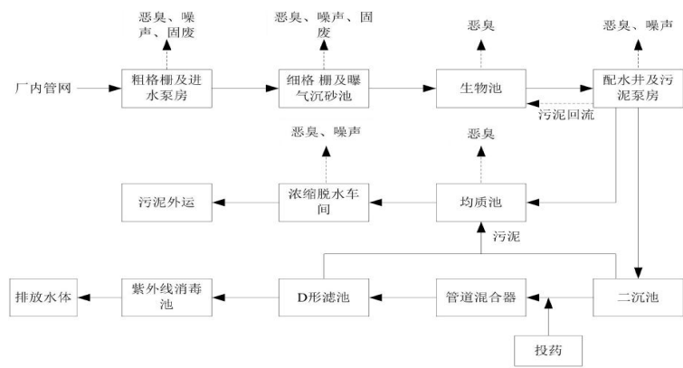
图 4. 杜阮污水处理厂污水处理工艺
