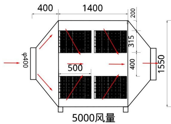
图 5. 活性炭箱设计图
