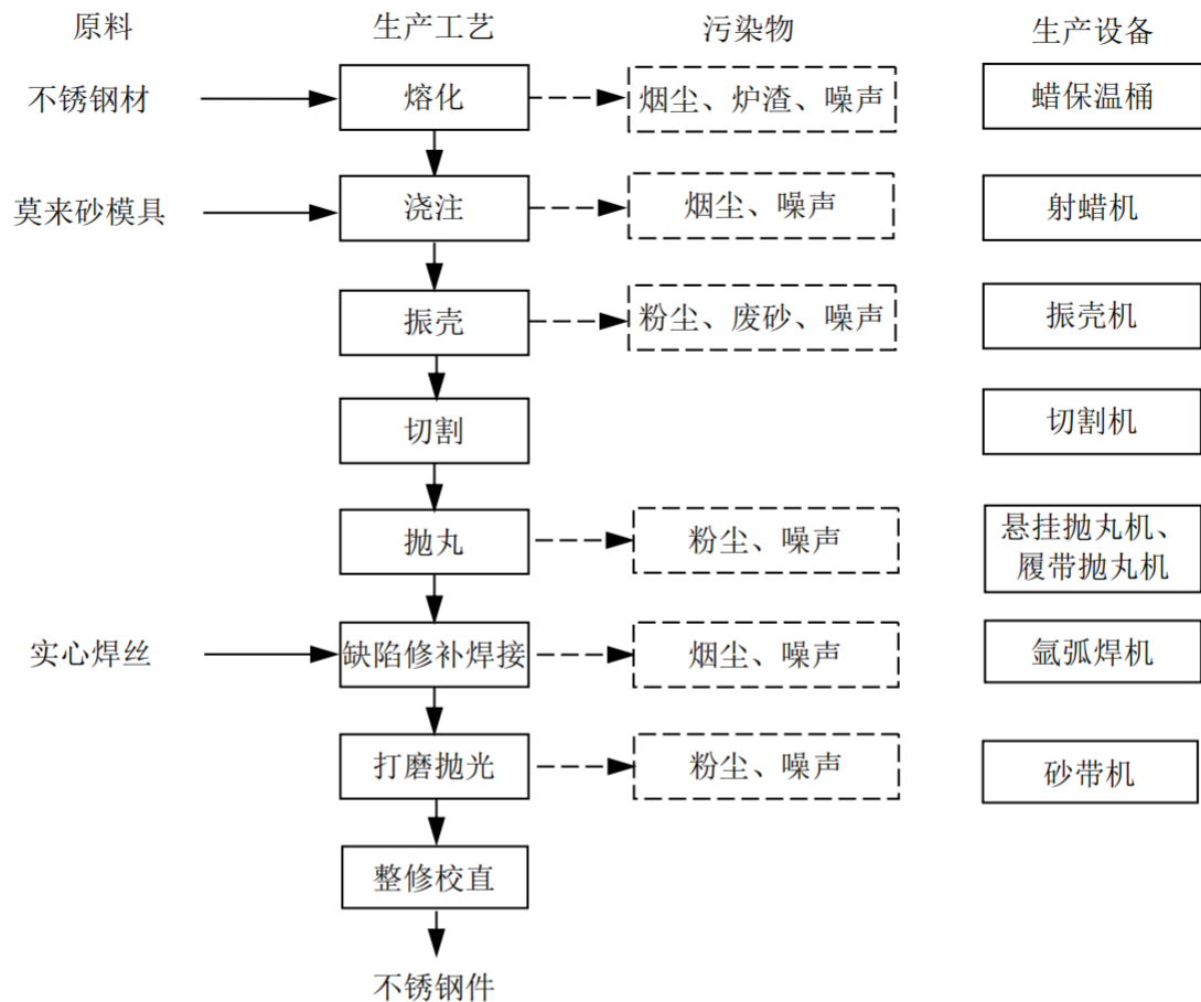
图 2-2 不锈钢件生产工艺流程图
