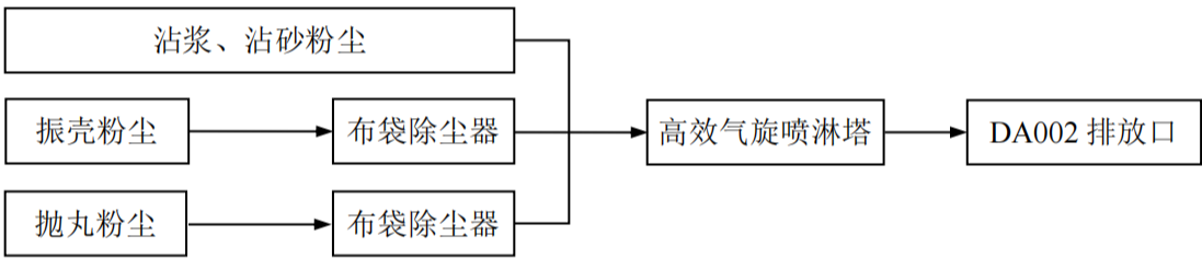
图 4-1 项目各粉尘废气处理流程图
